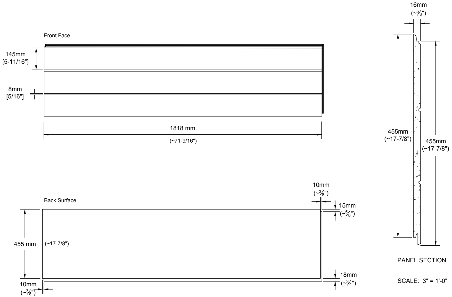
NICHIHA LATURA 1818 PANEL DETAIL SCALE: 1" = 1'-0"
